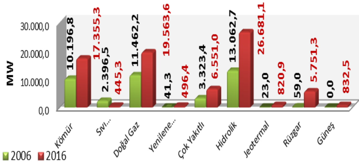
Grafik. 2. Türkiye'nin birincil enerji kaynaklarına göre 2006, 2016 kurulu gücü. Kaynak TEİAŞ
